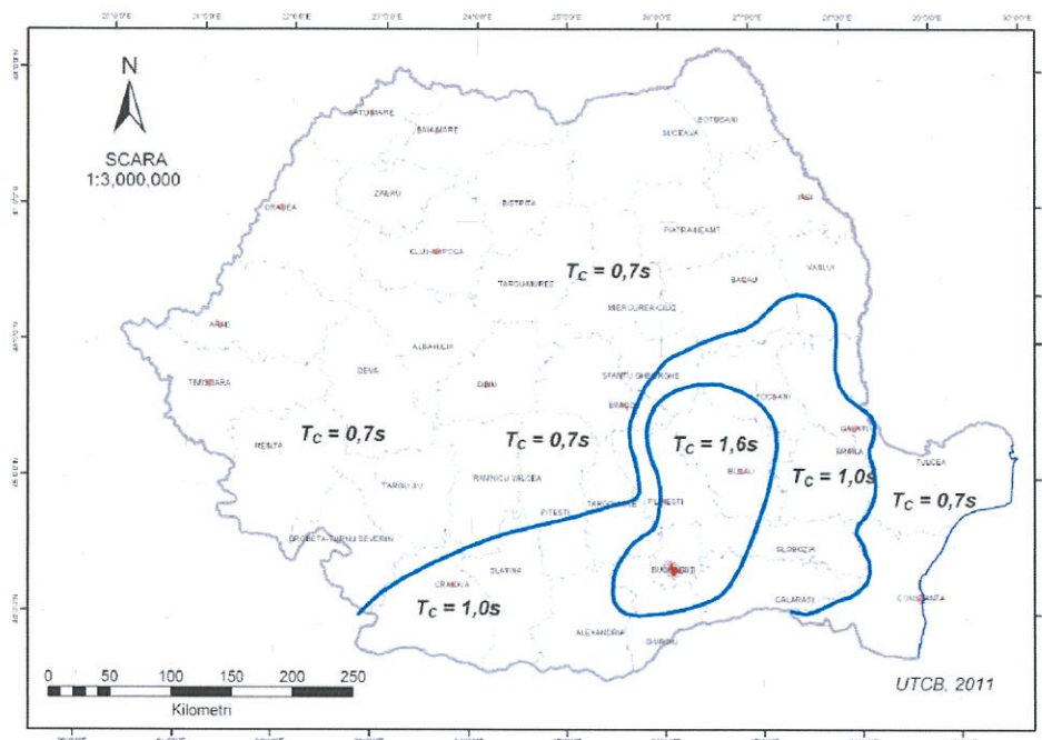
Perioada de control (colț), T_c pentru proiectare
