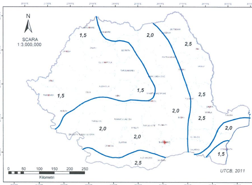
Zonarea valorilor caracteristice ale încărcării din zăpadă la sol s_k , în \text{kN/m}^2 și pentru altitudini A \leq 1000\text{m}
