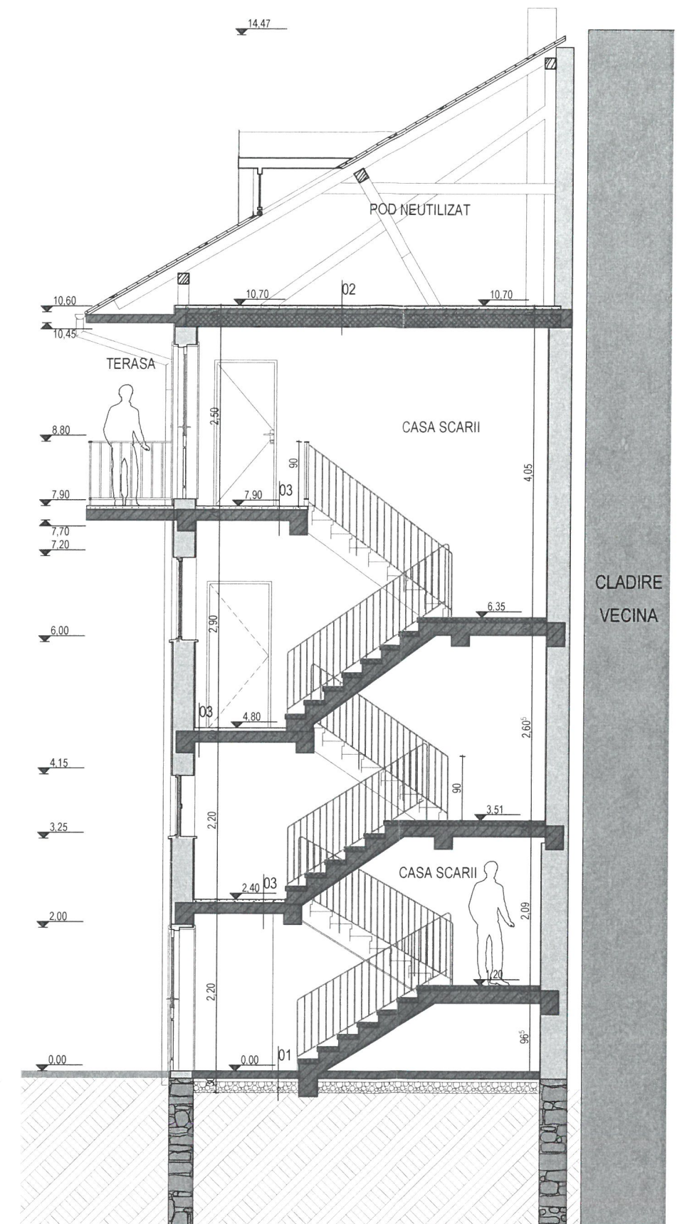
SECTIUNE TRANSVERSALA B-B, SC. 1:75
