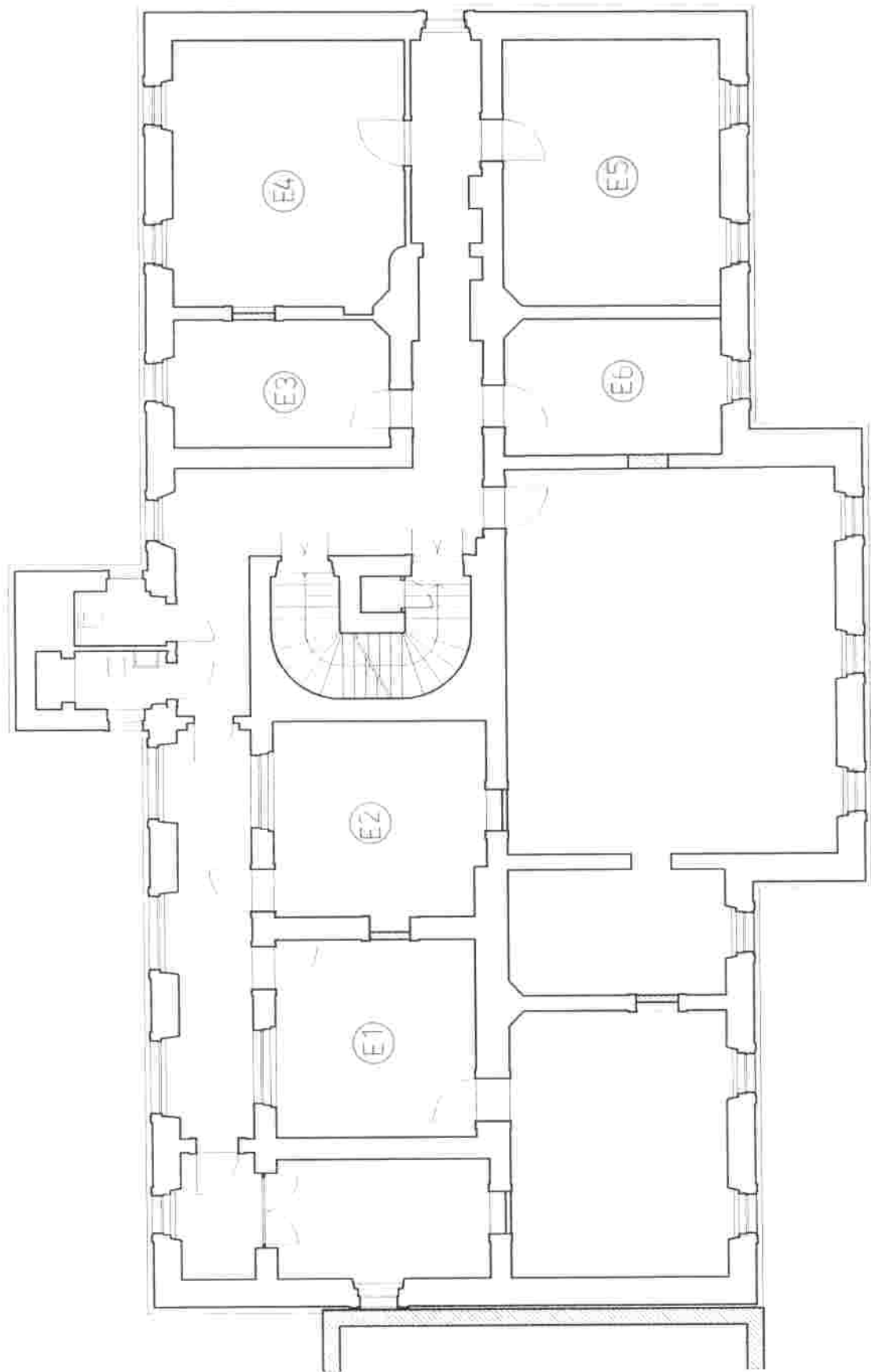
casa cu arcade etaj sc. 1:100
